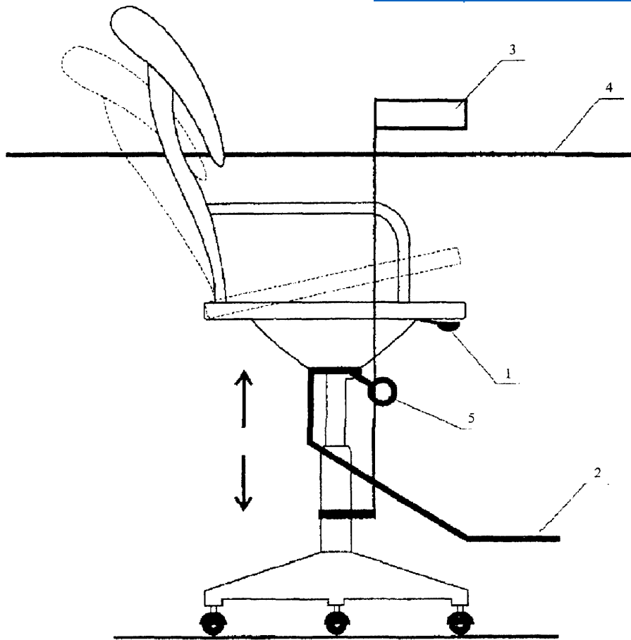
1 - ручное управление изменением высоты и углом наклона сиденья; 2 - подставка для ног; 3 - приспособление для рабочих инструментов; 4 - уровень рабочего стола; 5 - подъемный агрегат
