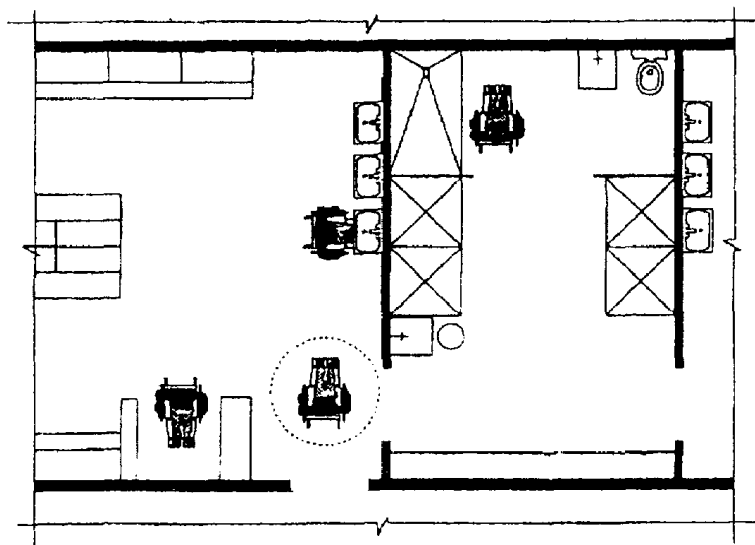
Размещение гардеробной (а) и душевой (б) для инвалидов
